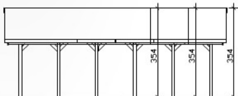
Seitenansicht
