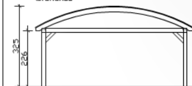
Vorderansicht
