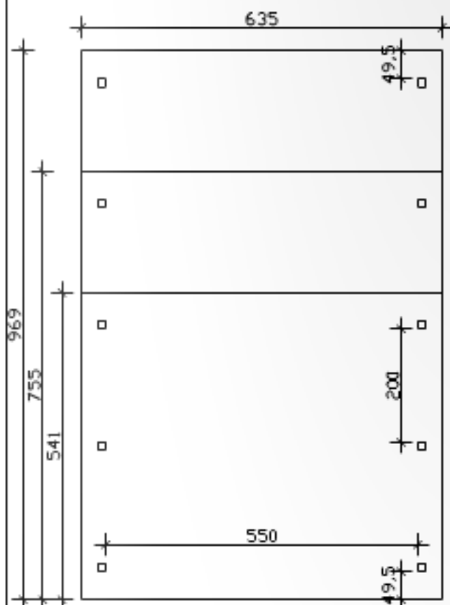
Grundriss
