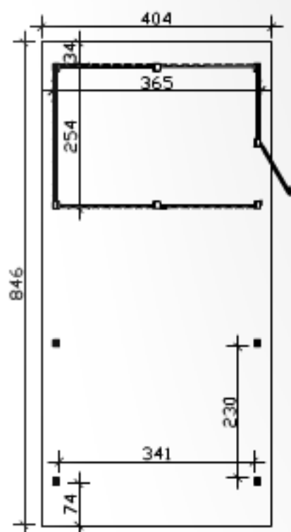
Grundriss
