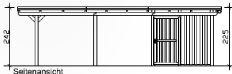
Seitenansicht
