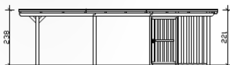
Seitenansicht
