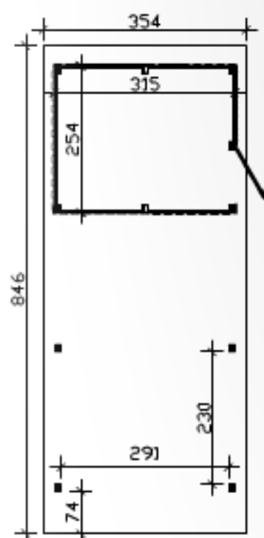
Grundriss
