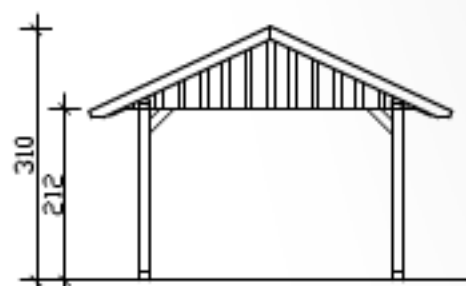
Vorderansicht
