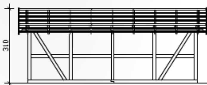
Seitenansicht
