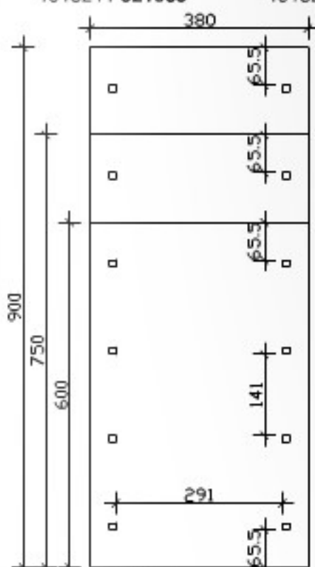
Grundriss
